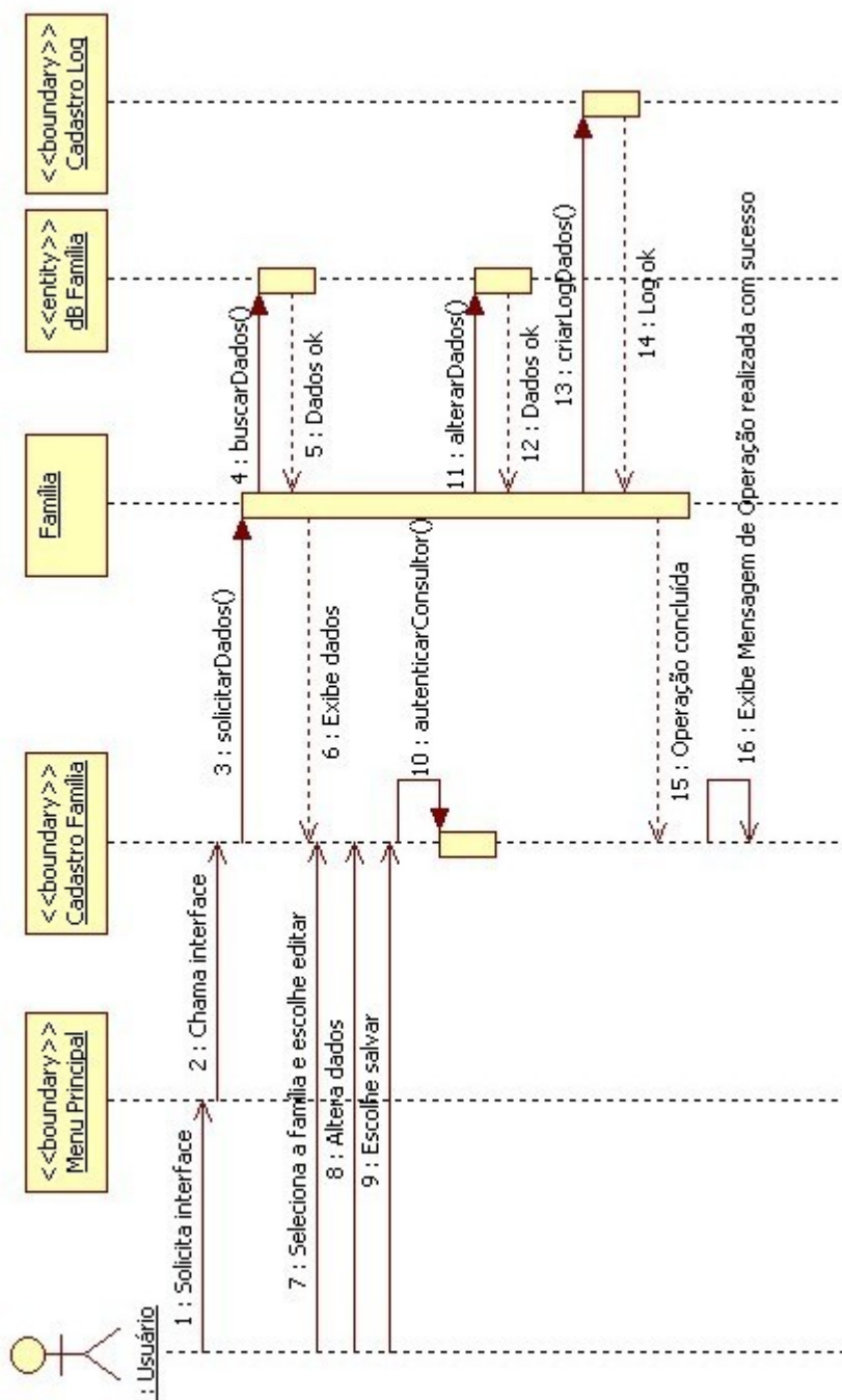
Figura 38 – Diagrama de Sequencia: Alterar Frequência Família
