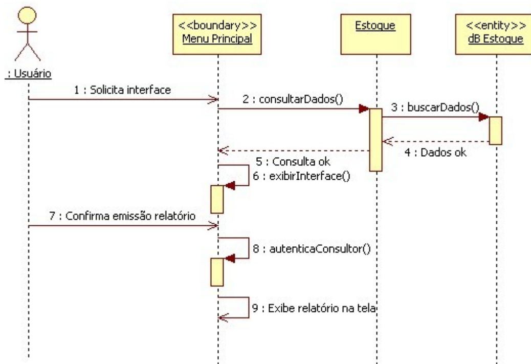
Figura 28 – Diagrama de Sequencia: Relatório de Vencimentos Estoque
